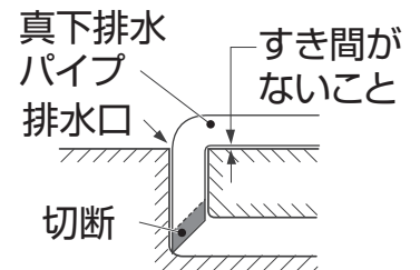
(洗濯機側面)
